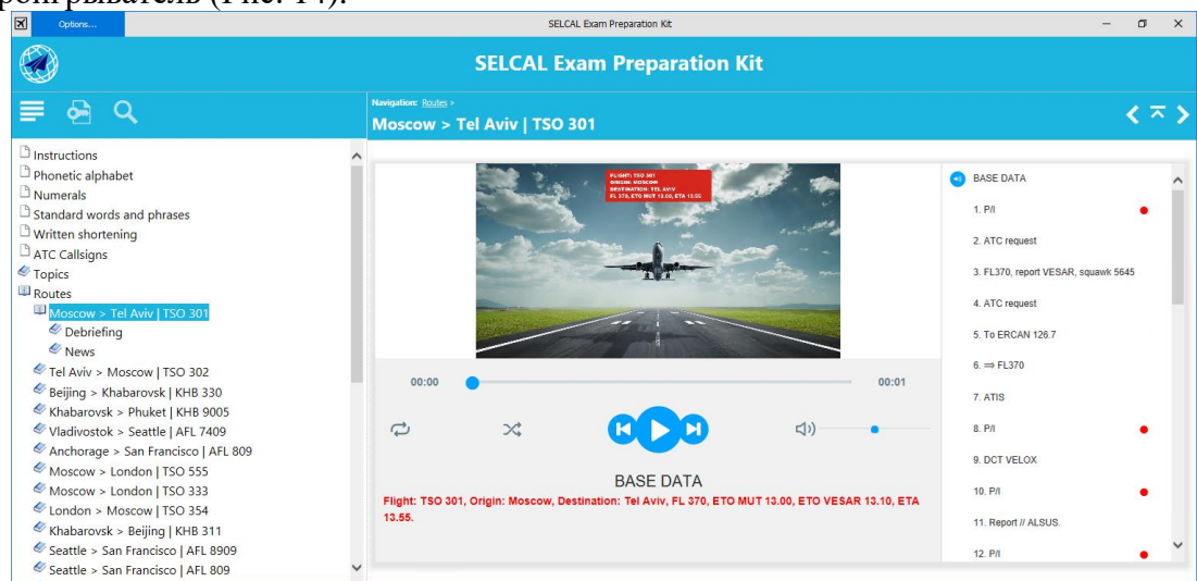
Рис. 14. Проигрыватель мультимедийных материалов
